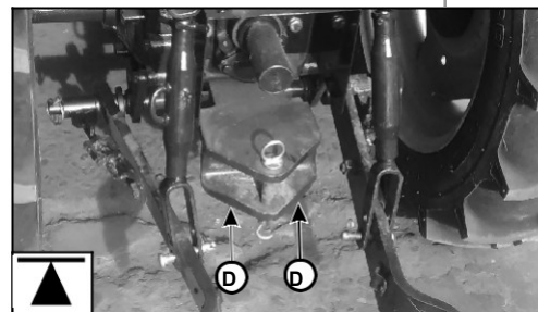
Kuva 5.23c - Traktorin etupään nostaminen
