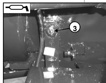
3. Kytkimen käyttöakseli
