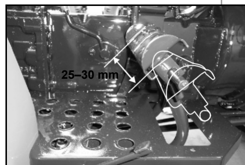
Kuva 5.10a: Malli 20
