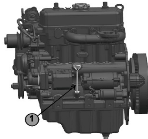
Kuva 5.3b: ITL-moottori
