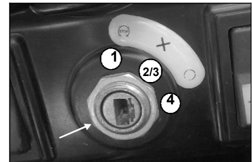
Kuva 4.3.1b - Käynnistyskytkin mallissa 22, 26 ja 30
