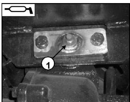
1. Keskitystappi
