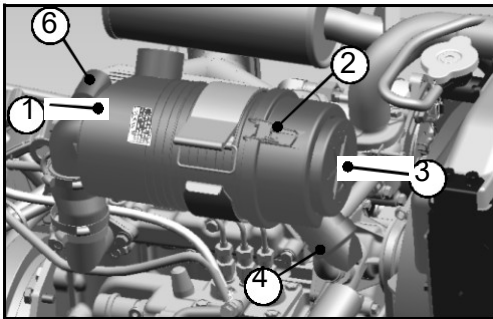
Kuva 5.8b: Mallit 22, 26 ja 30
