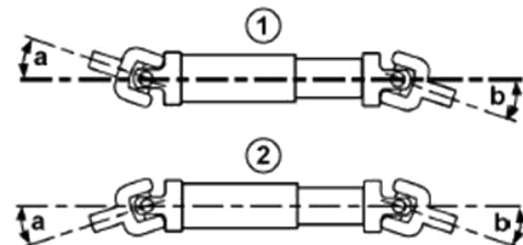
Nivelakselin nivelet
