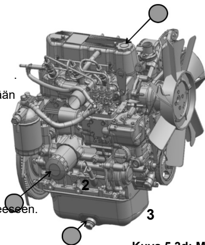
Kuva 5.3d: MHI-moottori
